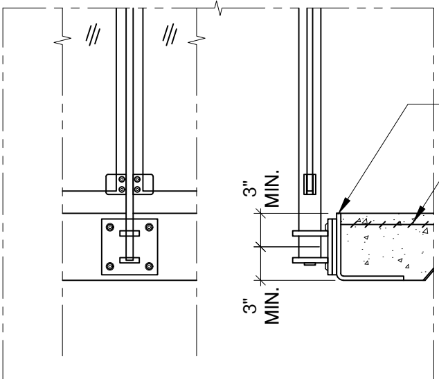
Welded @ Pour Stop - $$ Detail# BE-F05
